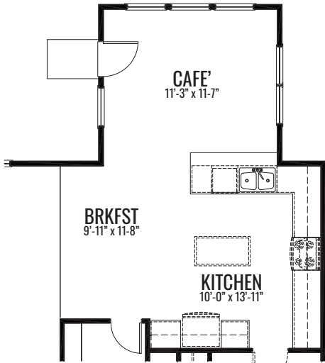
OPTIONAL CAFE'
