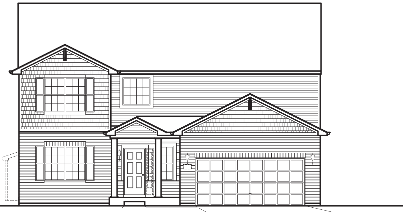
ELEVATION "C"
